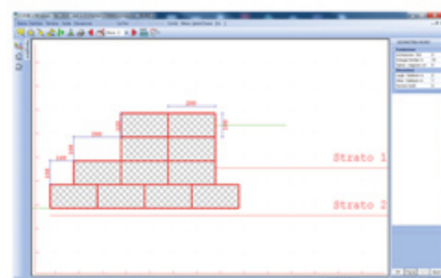
Input muro a Gabbioni
