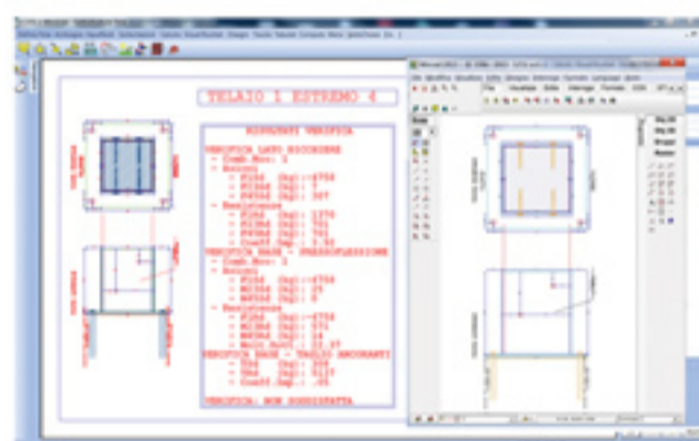
Colonna con bicchere di fondazione
